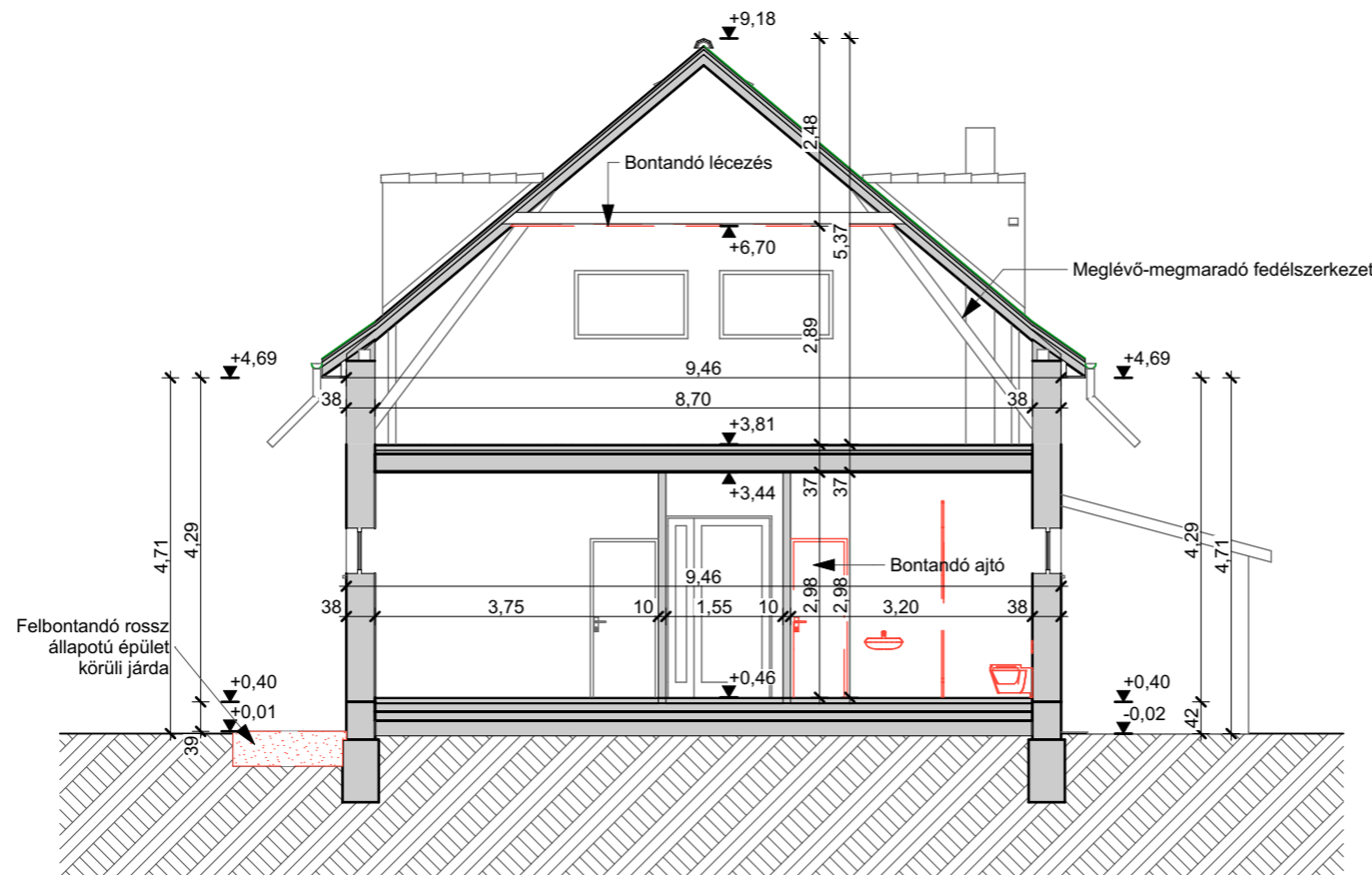
B - B metszet
