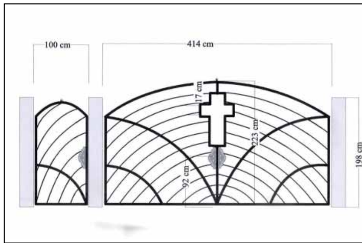
A temető kapujának látványterve
